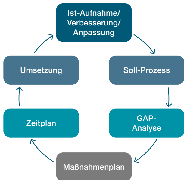
Abb. 2: Rechnungseingangsprozesse
